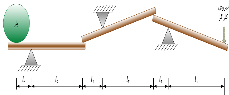
شکل ۱. اهرم مرکب
